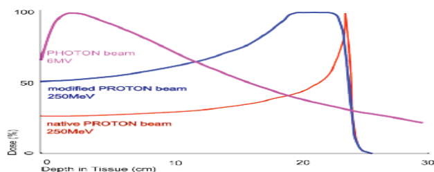
Figur: Det som utmärker protonstrålens egenskaper i jämförelse med vanlig fotonstrålning är att den huvudsakliga dosen avges samtidigt (röd kurva).
